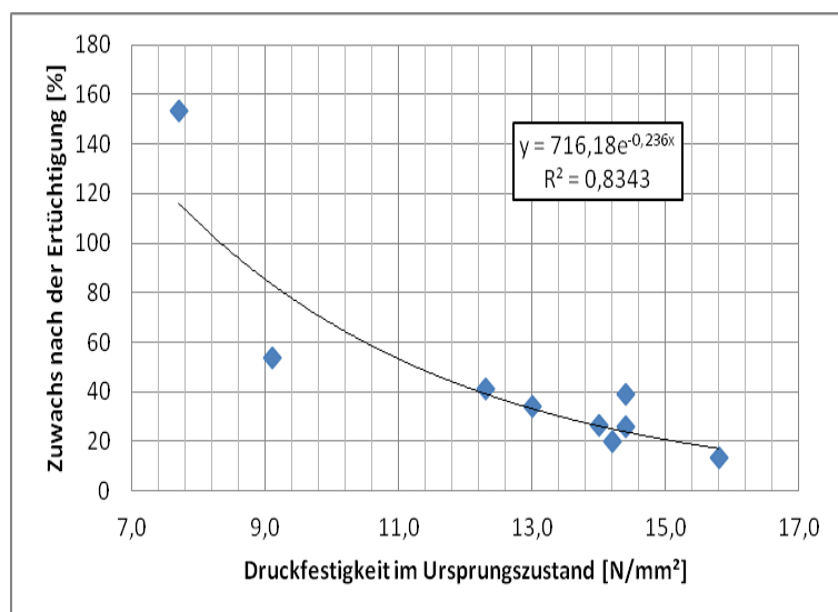
Abb. 2: Ertüchtigung
