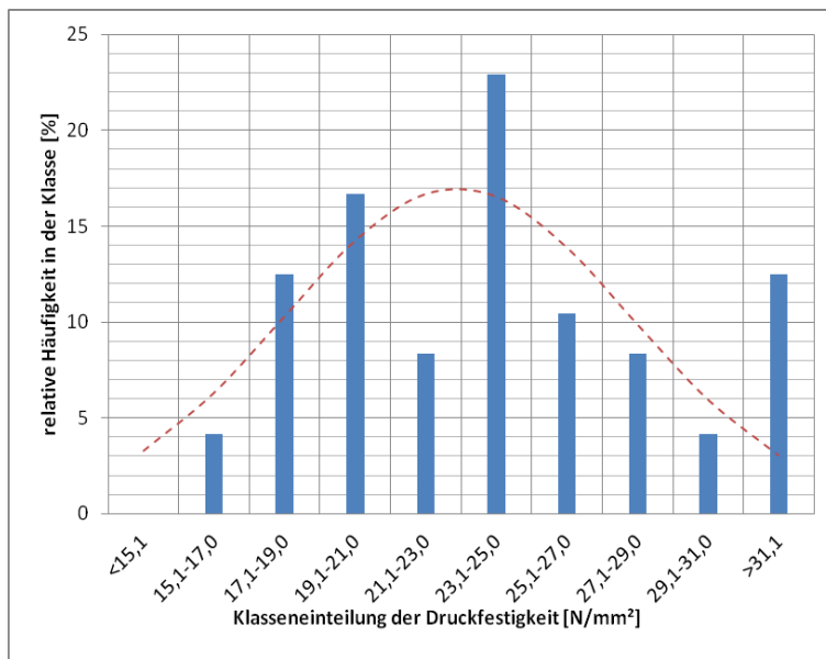
Abb. 3: Histogramm
